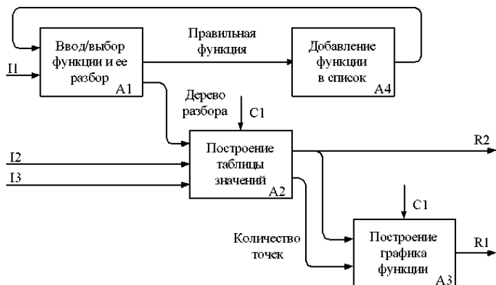
Рисунок 4 - Функциональные диаграммы
