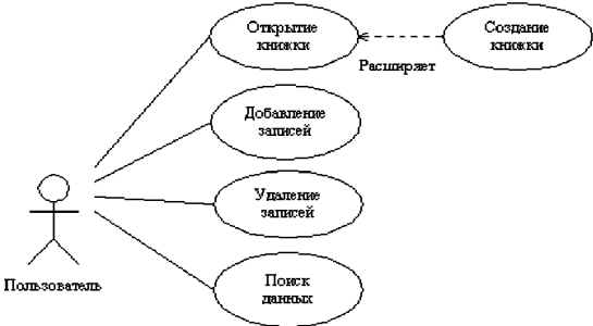
Рисунок 2 - Диаграмма вариантов использования
