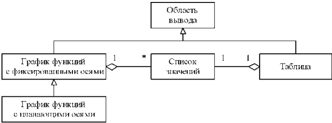
Рисунок 3 - Концептуальная диаграмма классов
